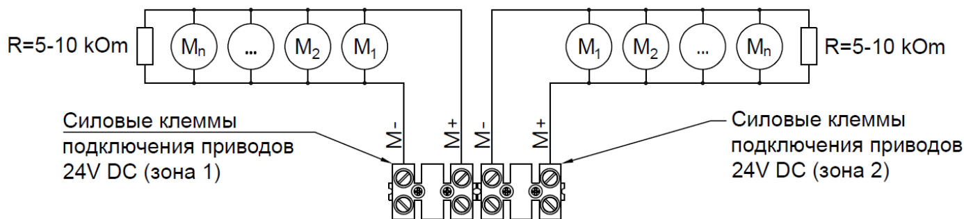
Рис. 4. Схема подключения приводов 24V DC
