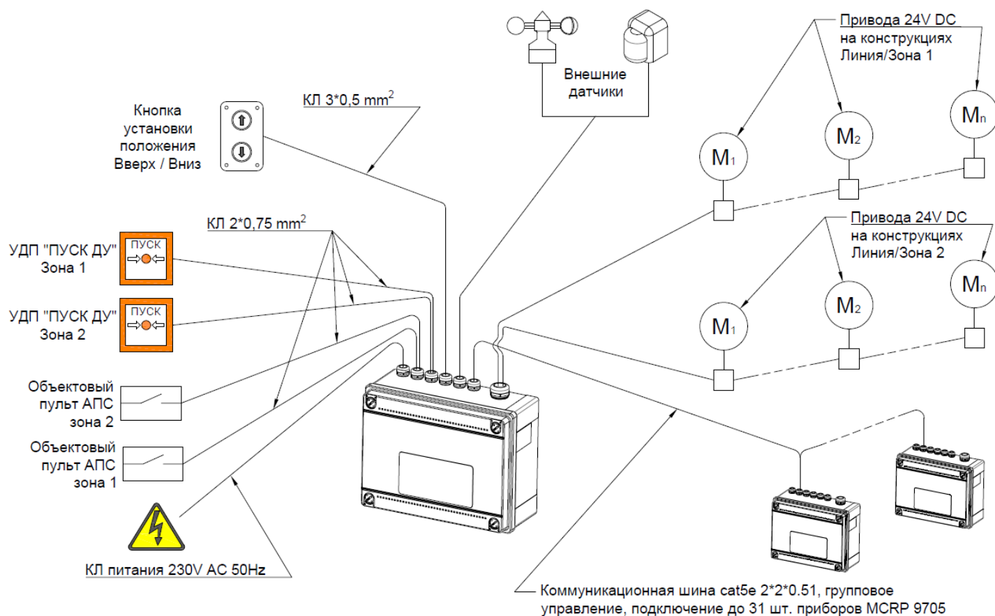
Рис. 3. Схема прокладки кабельных линий
