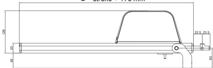
Actuator dimensions
