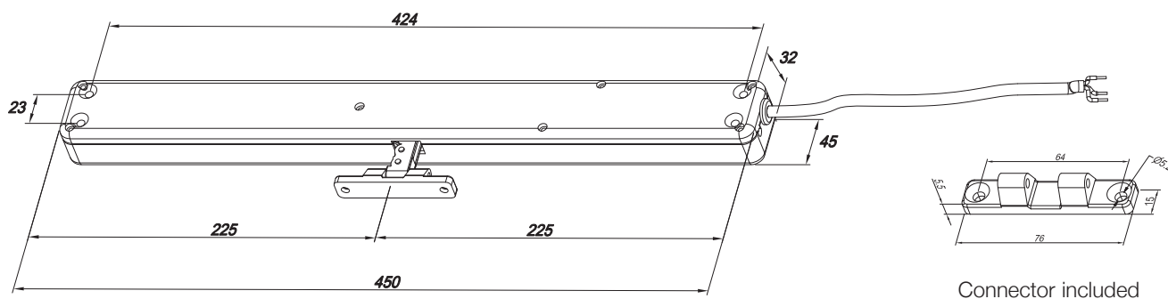
Actuator dimensions
